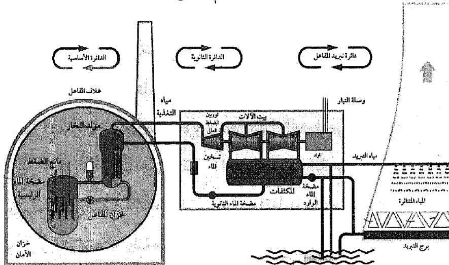
محطة قوى نووية تستخدم مفاعل الماء المضغوط
