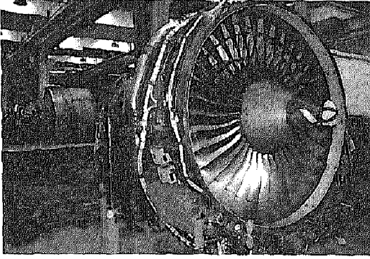
الشكل 35.1: مروحة توربو
