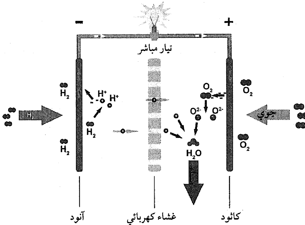
الشكل 13.10: مبدأ تشغيل خلية وقود
