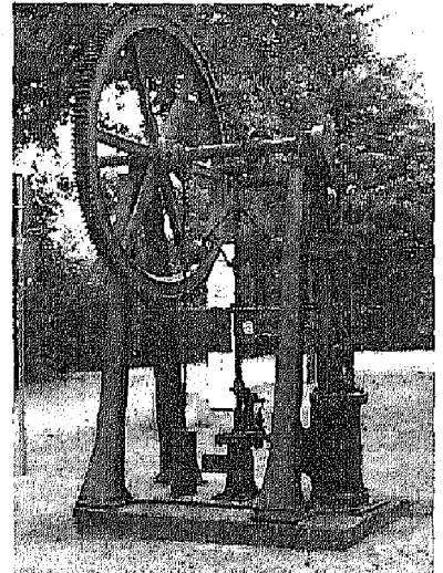
الشكل 24.6: آلة بخارية
