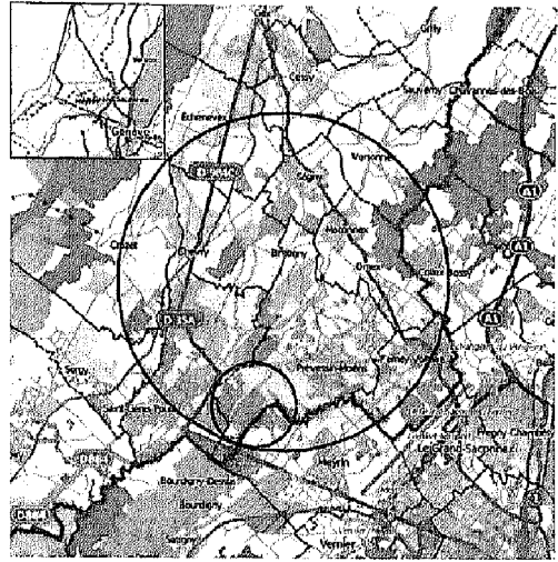
الشكل 48.6: لارج هادرون
