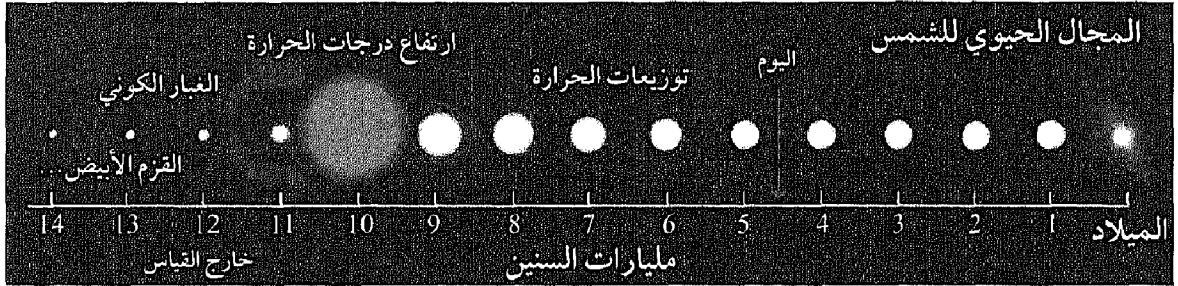
الشكل 2.2: نظام حياة الشمس
