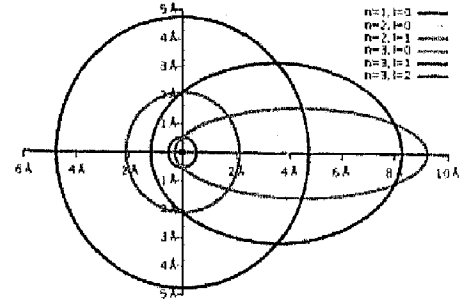
الشكل 5.5: النموذج الذري بوهر- زومرفيلد
