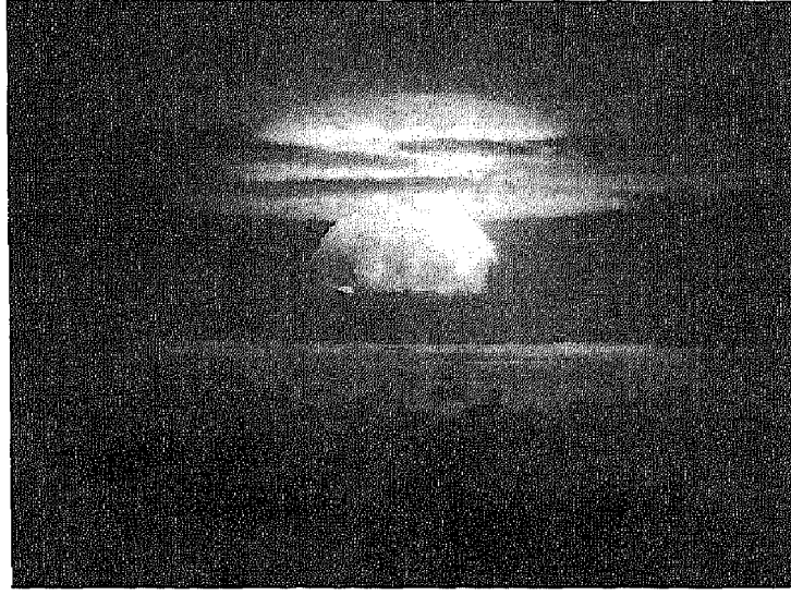
الشكل 5.10: تفجير قنبلة هيدروجينية عام 1954
